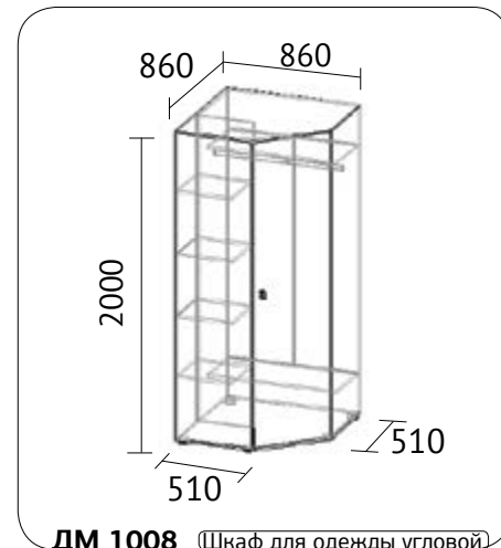
ДМ 1008 (Шкаф для одежды угловой)
