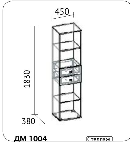
ДМ 1004 (Стеллаж)
