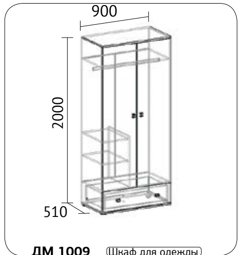
ДМ 1009 (Шкаф для одежды)
