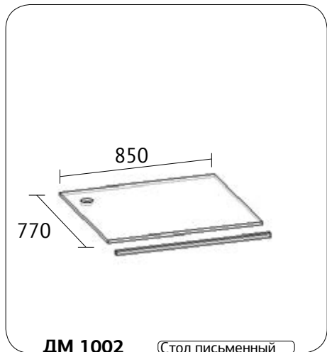
DM 1002 (Стол письменный)
