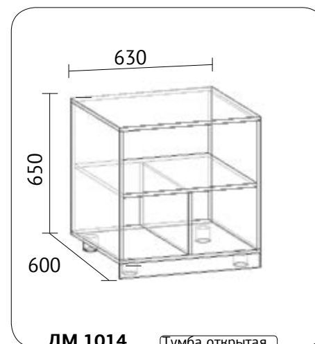
ДМ 1014 (Тумба открытая)
