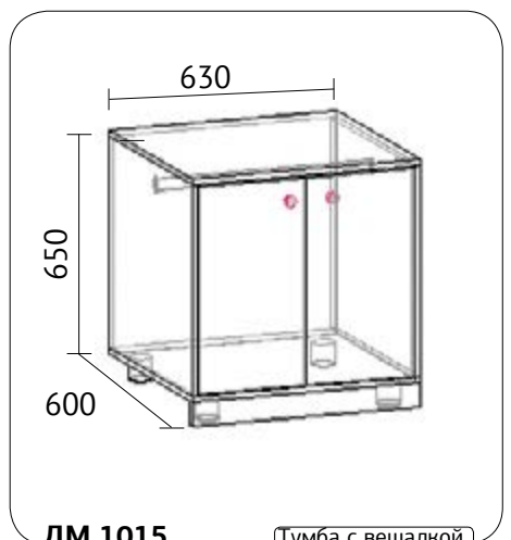
ДМ 1015 (Тумба с вешалкой)
