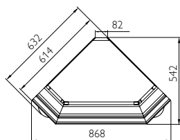
шкаф для посуды (угловой) ГМ 5260 (С), -01, дуб 2074 × 868 × 542
